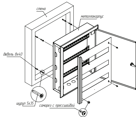
Рис. 1. Схема монтажа
