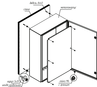
Рис. 1.1 - Схема настенного монтажа
