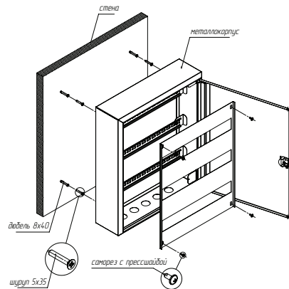
Рис. 1 - Схема монтажа
