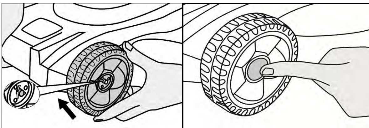
Рис. 2. Установка колес при креплении шплинтом
