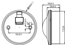
Рис. 3 - Габаритные и установочные размеры MS-25B накладного исполнения
