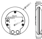
Рис. 1 - Габаритные и установочные размеры MS-24B
