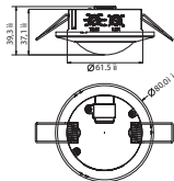
Рис. 2 - Габаритные и установочные размеры MS-25B встраиваемого исполнения
