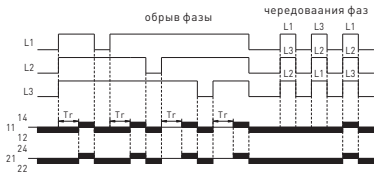
Рис. 1 – Работа реле при обрыве фазы и неверной последовательности фаз
