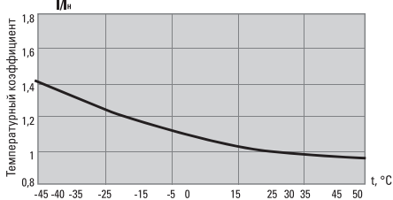
Рис. 2 Температурный коэффициент
