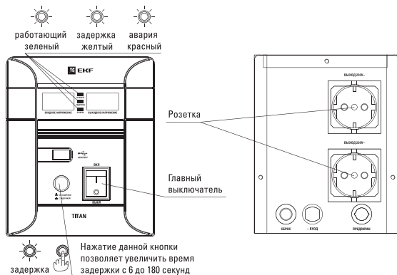
Рис. 3 Внешний вид стабилизатора F-1500-2000
