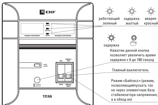
Рис. 4 Внешний вид стабилизатора F-3000-5000
