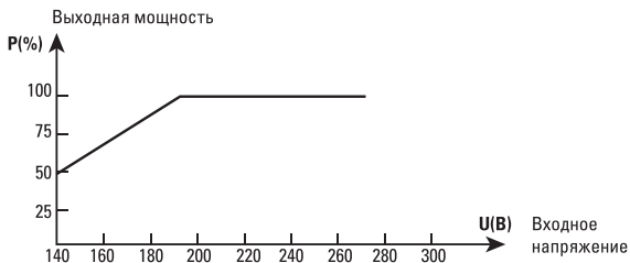
Рис. 1 График зависимости выходной мощности от входного напряжения
