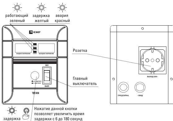
Рис. 2 Внешний вид стабилизатора F-500-1000
