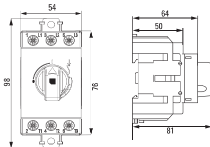
Рис. 1б Габаритные размеры рубильника MS 63А
