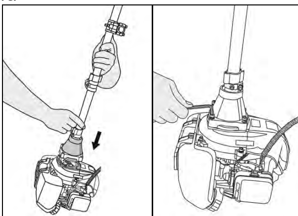
Рис. 6. Установка штанги
