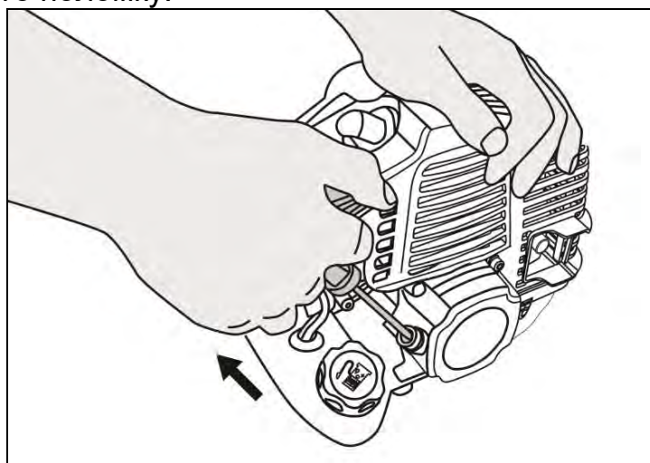
Рис. 23. Запуск двигателя
