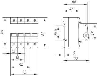
Рис. 1 Габаритные и установочные размеры ВН-29
