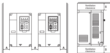
Монтажная схема верхнего устройства
