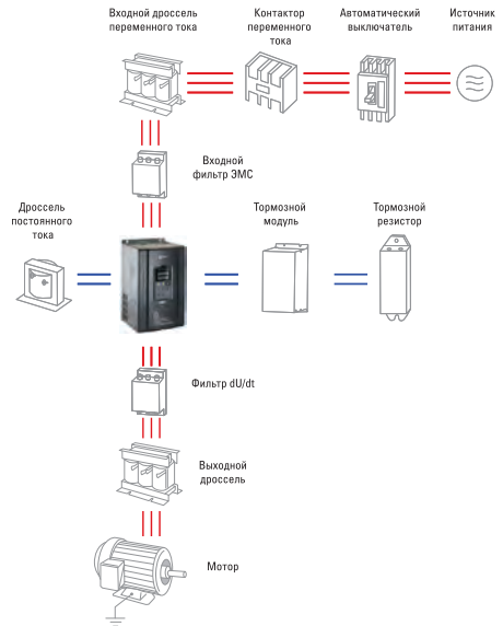
Рис. 11-1 Схема подключения периферийных устройств
