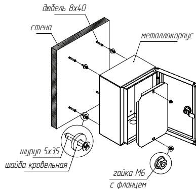
Рис. 1.1 - Схема настенного монтажа
