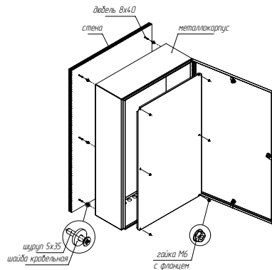
Рис. 1.1 - Схема настенного монтажа
