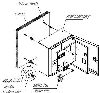
Рис. 1.1 - Схема настенного монтажа
