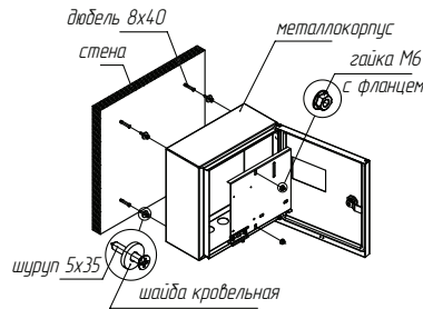
Рис. 1.1 - Схема настенного монтажа
