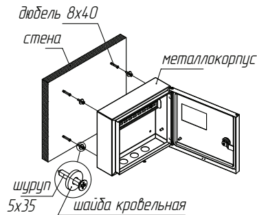
Рис. 1.1 - Схема настенного монтажа
