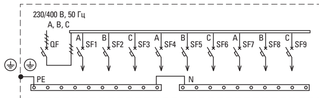
Рис. 1 - Схема подключения
