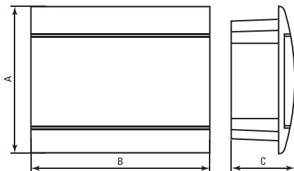
Рис. 1 Габаритные размеры щитов SlimBox
