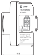
Рис. 15 Габаритные и установочные размеры
