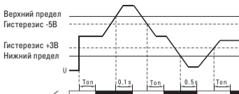
Рис. 1 Диаграмма напряжения реле
