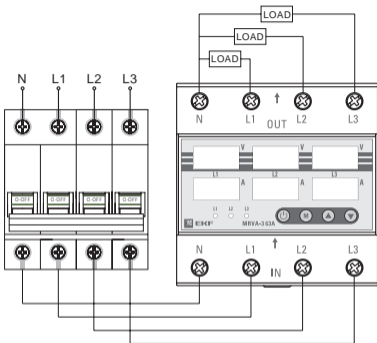
Рис. 14 Схема подключения
