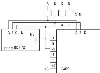
Рисунок 2. Схема подключения с применением реле контроля фаз
