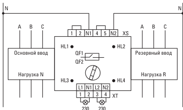
Рисунок 1. Схематичное изображение лицевой панели АВР МСВ
