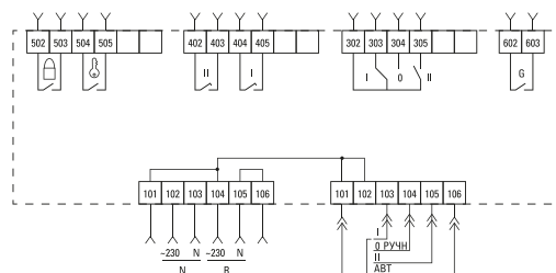
Схема подключения внешних проводников для АВР ТСП1 от 125 до 400 А
