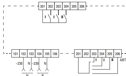
Схема подключения внешних проводников для АВР ТСП1 100 А
