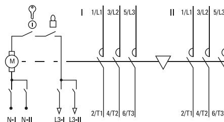
Схема подключения внешних проводников для АВР ТСП1 630 А
