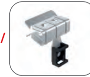
Зажим балочный 3-8/8-14 мм под нейл. стяжку ZB3-8-S/ZB8-14-S
