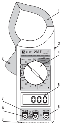
Рис. 1 Элементы лицевой панели
