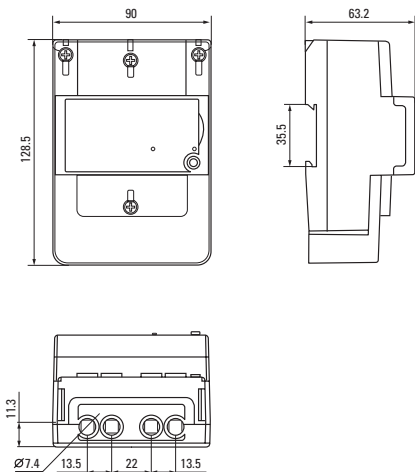
Рисунок 3 – Габаритные размеры счетчика
