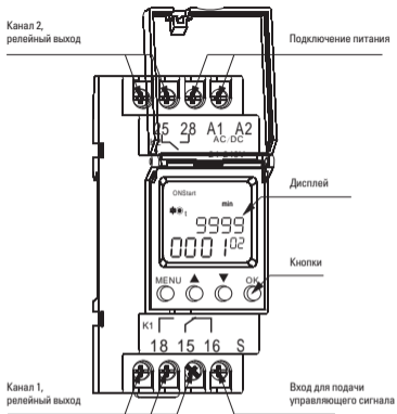
Рис.1 Таймер TM-24
