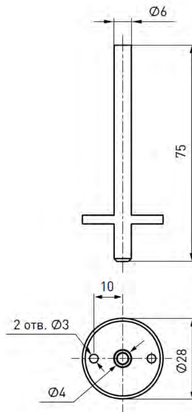
Штуцер
