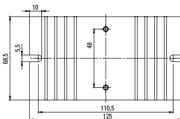
Рис. 2 Твердотельного реле 40А
