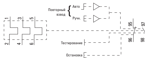
Рис. 3 – Принципиальная схема теплового реле РТЭ
