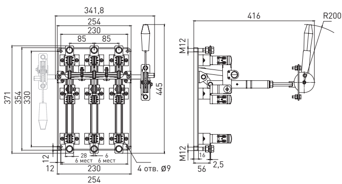
Рис. 7 - Габаритные и установочные размеры разъединителя типа РПС-400
