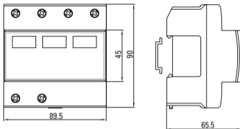
Рисунок 7 Габаритные и установочные размеры
