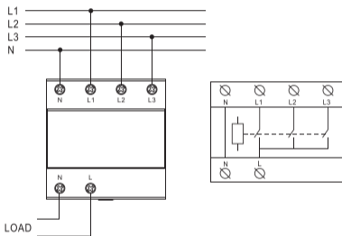
Рисунок 6 Схема подключения
