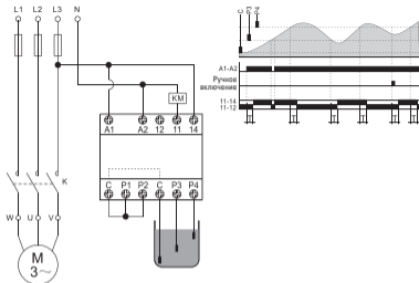
Рисунок 1. Одна емкость. Наполнение по 3 датчикам.
