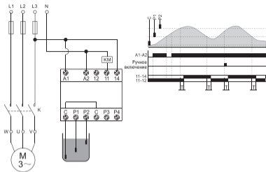
Рисунок 3. Одна емкость. Осушение по 3 датчикам
