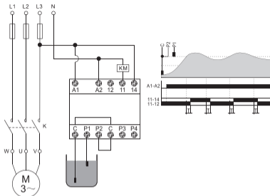
Рисунок 4. Одна емкость. Осушение по 2 датчикам
