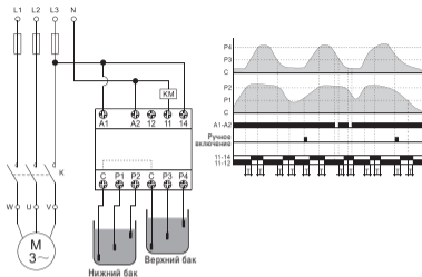
Рисунок 5. Две емкости по 3 датчикам
