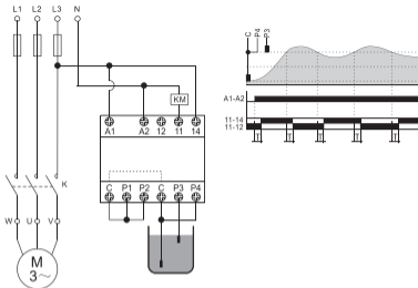
Рисунок 2. Одна емкость. Наполнение по 2 датчиком
