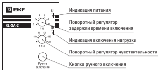
Рисунок 6. Панель управления.
