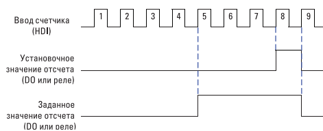
Схема функции отсчёта
