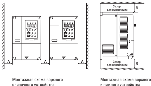
Рис. 4-1 Монтажная схема
