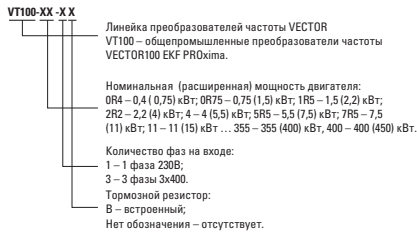
Рис. 2-1 Расшифровка номера преобразователя
