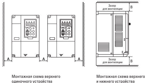
Рис. 4-1 Монтажная схема
