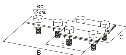
Зажим контрольный
