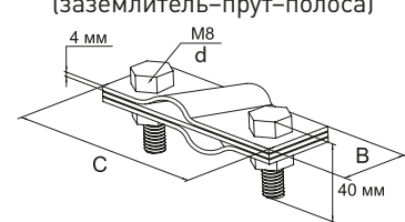
Зажим продольный
