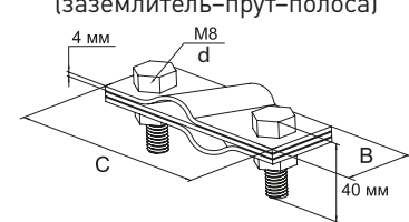
Зажим продольный
