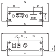
Рисунок 2-б – Габаритные и установочные размеры модема
