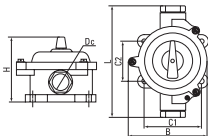
Рис. 9 Пакетные переключатели серии ПП – Исполнение в силовом корпусе
