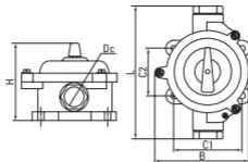
Рис. 5 Пакетные выключатели серии ПВ – Исполнение в силовом корпусе
