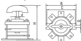
Рис.1 Пакетные выключатели серии ПВ – Исполнение 3
