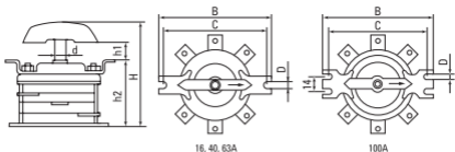
Рис. 7 Пакетные переключатели серии ПП – Исполнение 1
