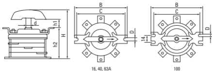
Рис. 2 Пакетные выключатели серии ПВ – Исполнение 1
