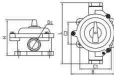
Рис. 5 Пакетные выключатели серии ПВ – Исполнение в силовом корпусе
