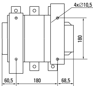
КТЗ -630 А
