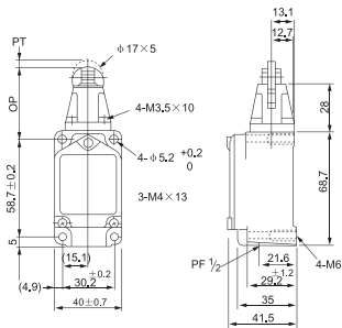
Рис. 7 Габаритные размеры концевых выключателя WLD2 EKF PROxima
