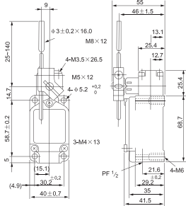
Рис. 4 Габаритные размеры концевых выключателя WLCL EKF PROxima
