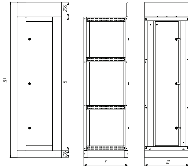
Рис.1 - Общий вид шкафов ЩО-70 Unit
