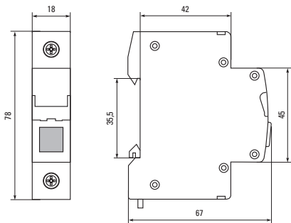
Рисунок 1 – Габаритные размеры сигнальных ламп AV-L
