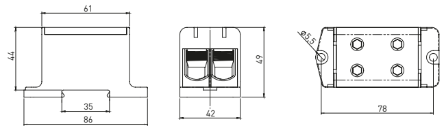
КСВ 16-95 (двойные)
