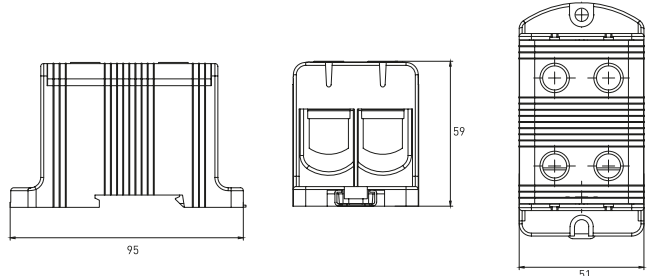
КСВ 16-50 (тройные)
