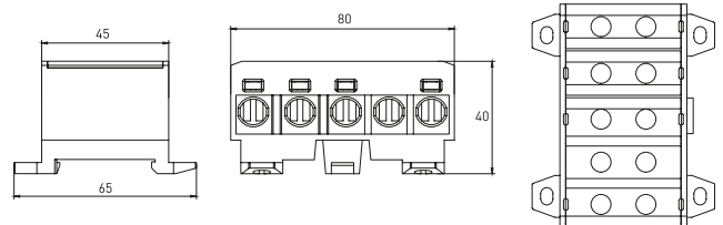
КСВ 2,5-35 (пятиполюсные)
