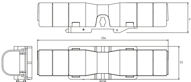
КСВ6 10-120
