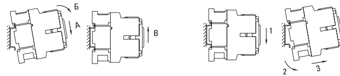
Монтаж, контактора, шаги: А, Б и В
